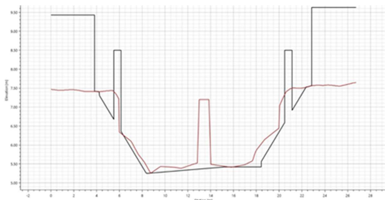
Figur 3 Rød strek viser eksisterende tverrsnitt, mens svart strek viser nytt tverrsnitt.
