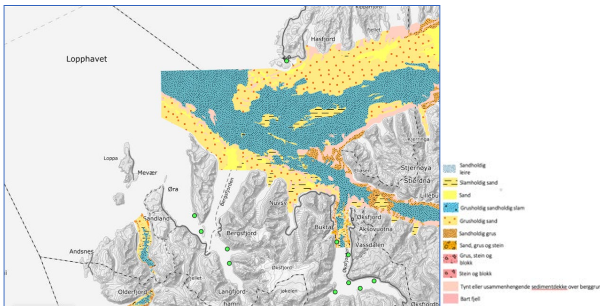
Fig. 6.1: Oversikt over bunnsedimenter (kornstørrelse) og akvakulturlokaliteter (grønn prikk) i Loppa.
